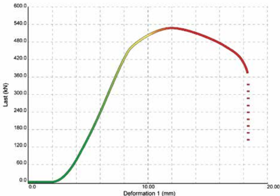
Last-deformationskurva från utfört prov enligt EN 15048-2
